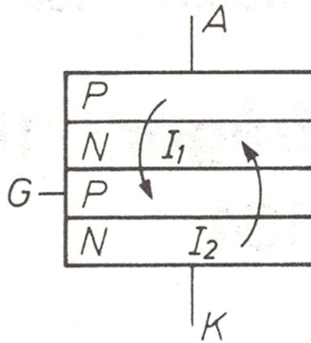
Tyristorkristall
